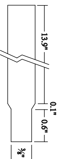
Aft Core Conduit
